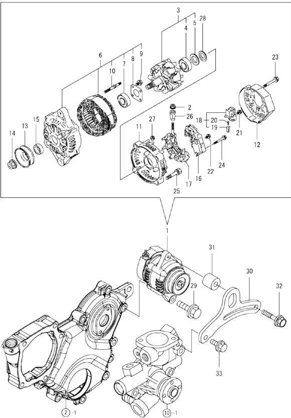
Fig.21. (18A)GENERATOR
