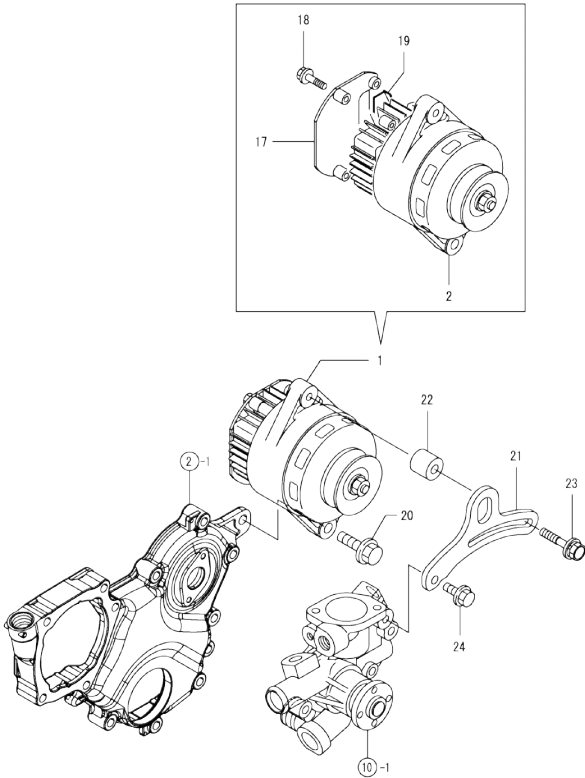
Fig.18. GENERATOR
